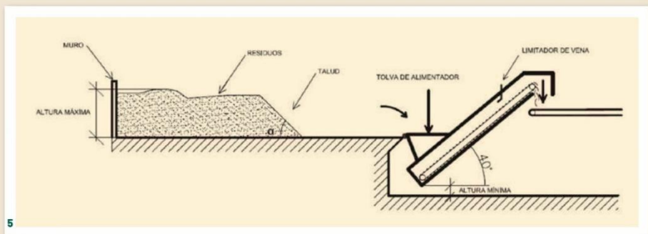
5. Alimentador empotrado en área de descarga.
