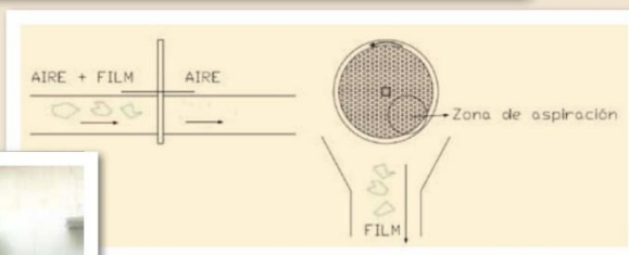
7. Sistema de separación mediante paso de corriente a través de malla circular giratoria.
