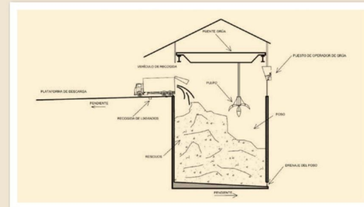
2. Foso de descarga.
