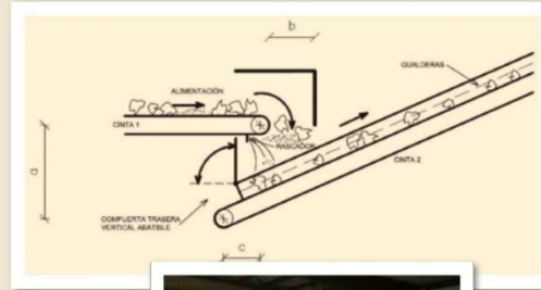
4. Tova de transvase entre cintas en línea.
