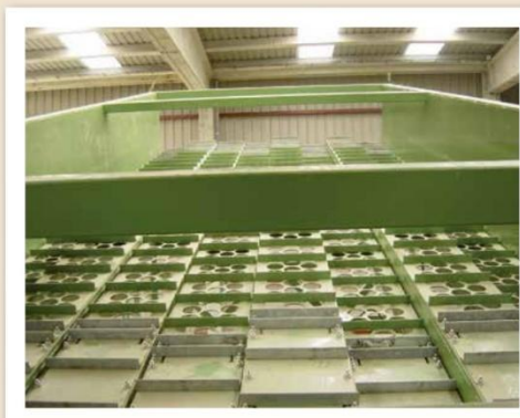
4. Pádeles del separador balístico.
