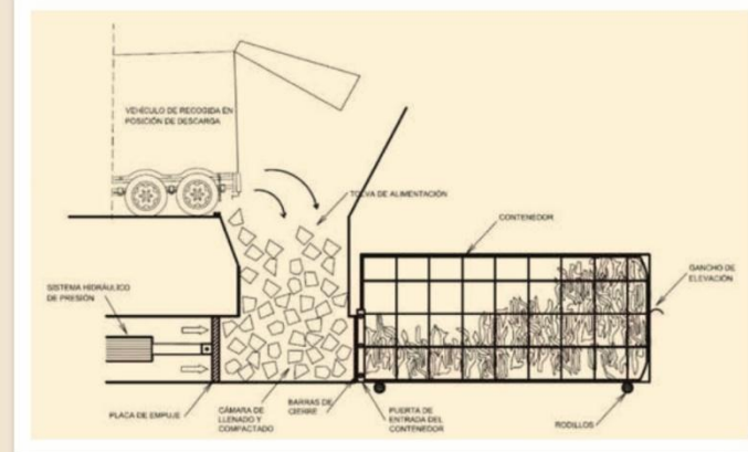
1. Compactadores estáticos.
