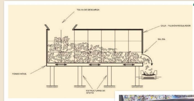
6. Alimentador de fondo móvil.
