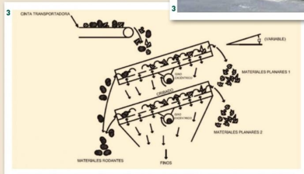
3. Separador balístico de dos grupos de pádeles de misma inclinación.
