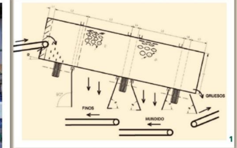
1. Trómel de dos mallas.
