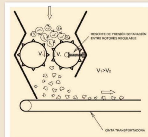
4. Abre-bolsas tipo triturador.
