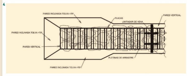
4. Alimentador de placas inclinado (planta).
