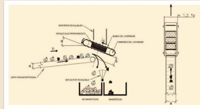
1. Over-band en línea.
