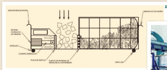
2. Contenedor auto-compactador.
