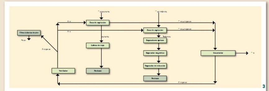
2. Sistema de aspiración con una boca de aspiración.
