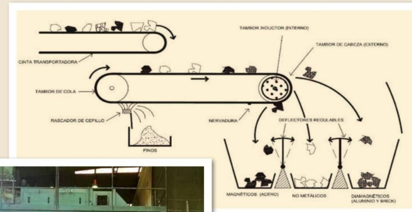
2. Separador de inducción.
