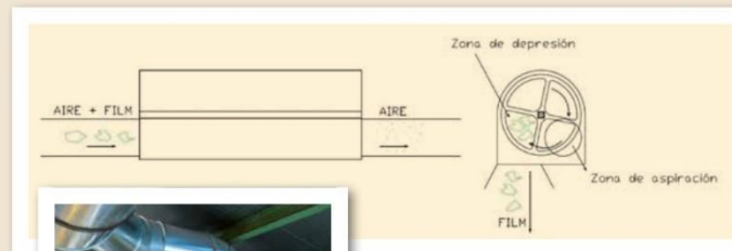
8. Sistema de separación mediante válvula alveolar.
