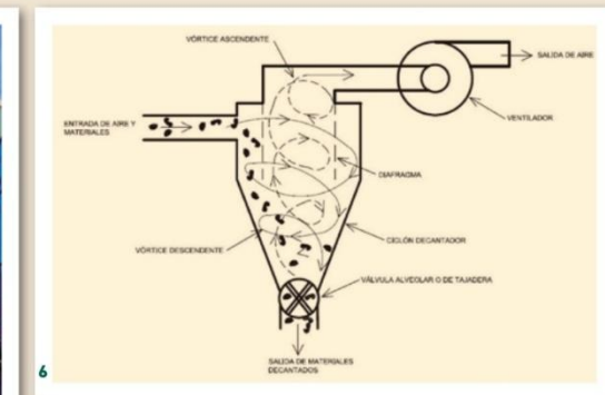
6. Sistema de separación mediante ciclón.
