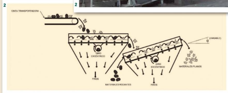
2. Separador balístico de rebote en dos planos.
